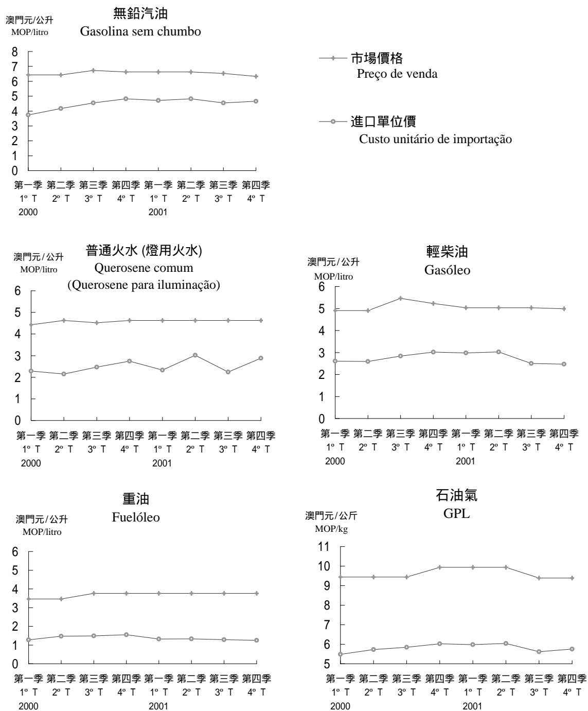
GRÁFICO 3 - EVOLUÇÃO DO CUSTO UNITÁRIO DE IMPORTAÇÃO E DO PREÇO DE VENDA DOS COMBUSTÍVEIS
